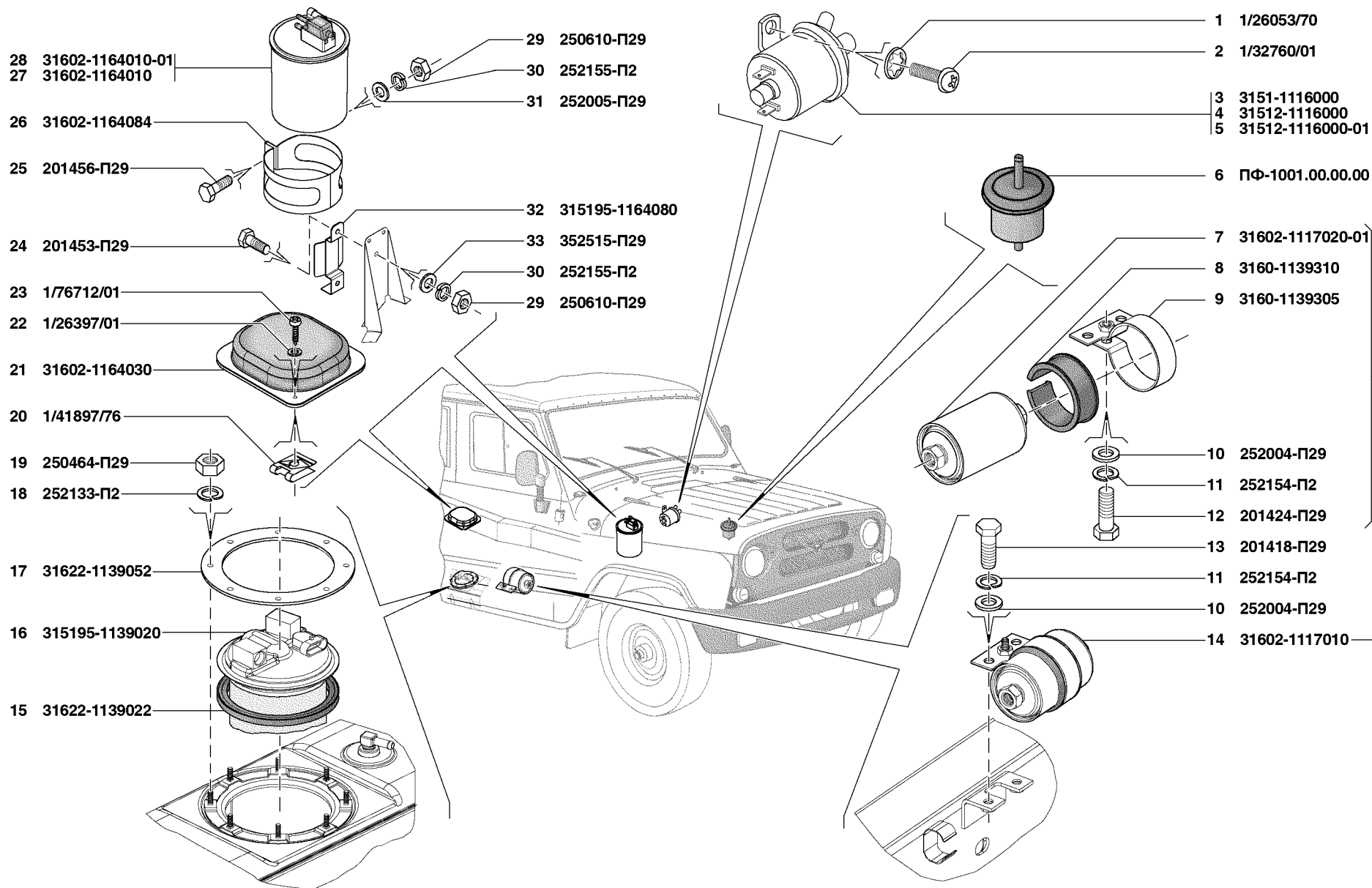
Рис. 37. Клапан топливный электромагнитный (1116), фильтр тонкой очистки топлива (1117), насос топливный низкого давления электрический (1139), система улавливания топливных испарений (1164) Fig. 37. Electromagnetic fuel valve (1116), fine fuel filter (1117), electric low-pressure fuel pump (1139), fuel fume catch system (1164)
